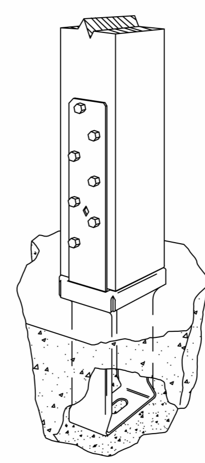
SIMPSON POST BASE CBSQ N.T.S.
